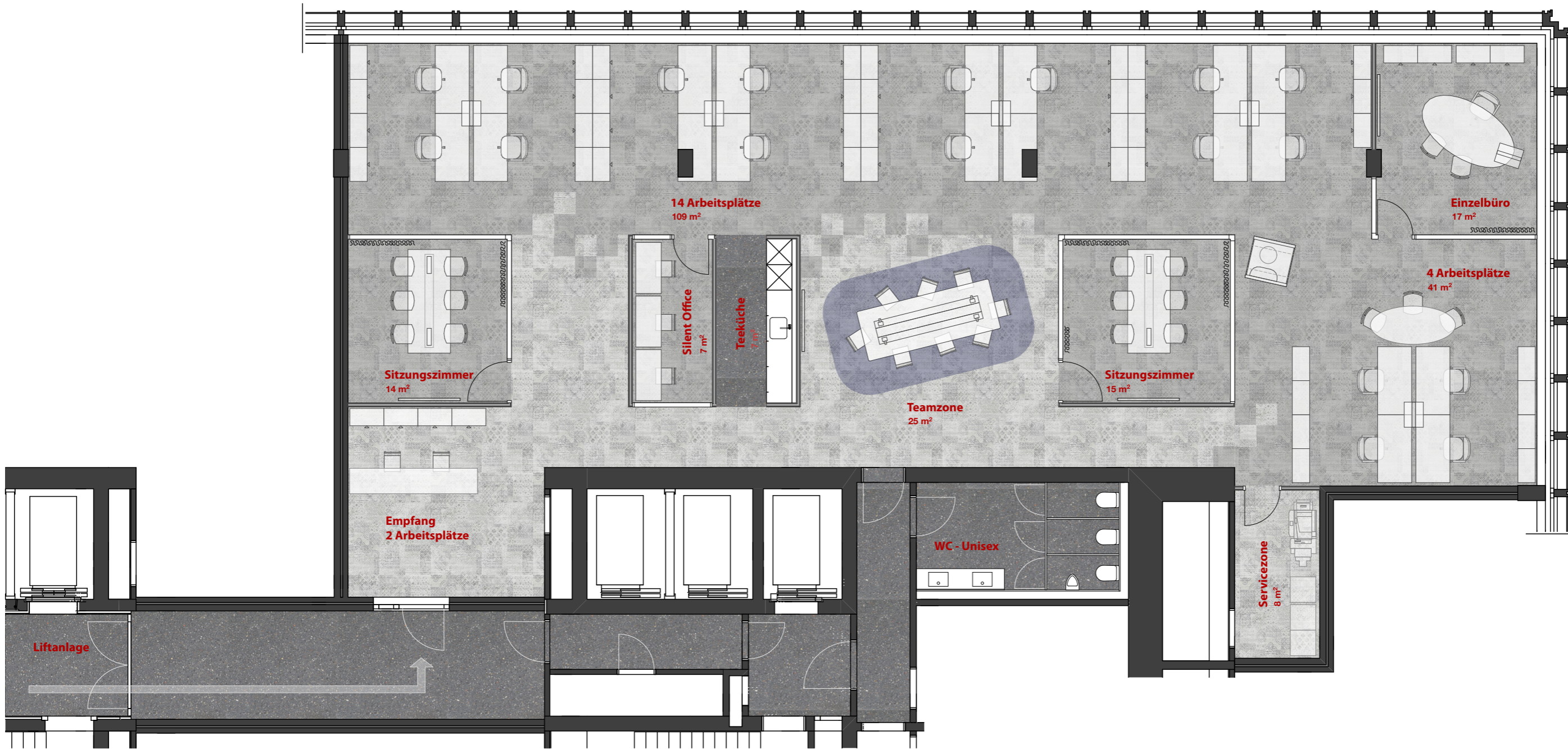
Grundrissausschnitt 1:100
